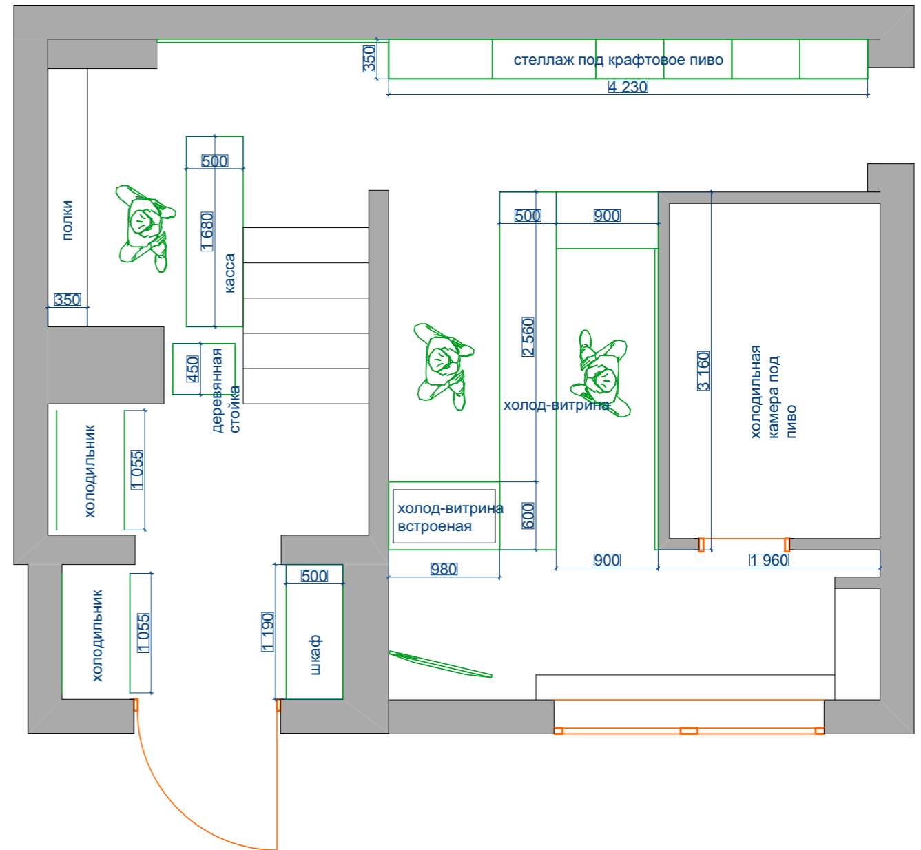
План расстановки мебели
