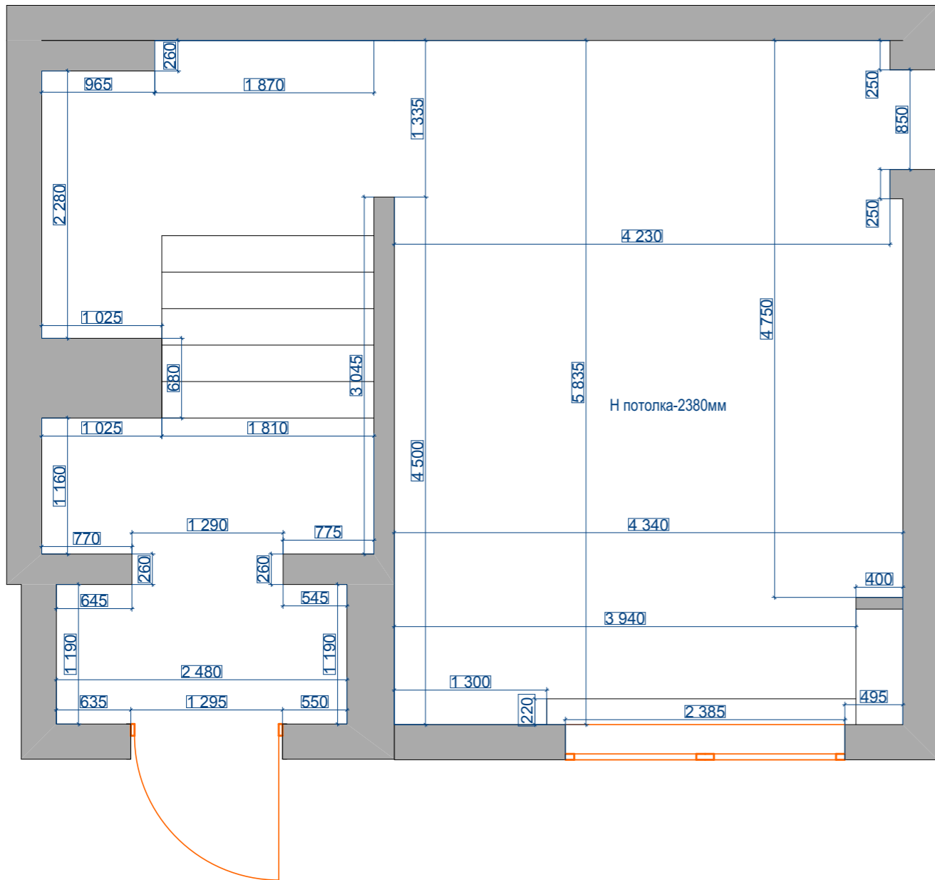
Обмерочный план
