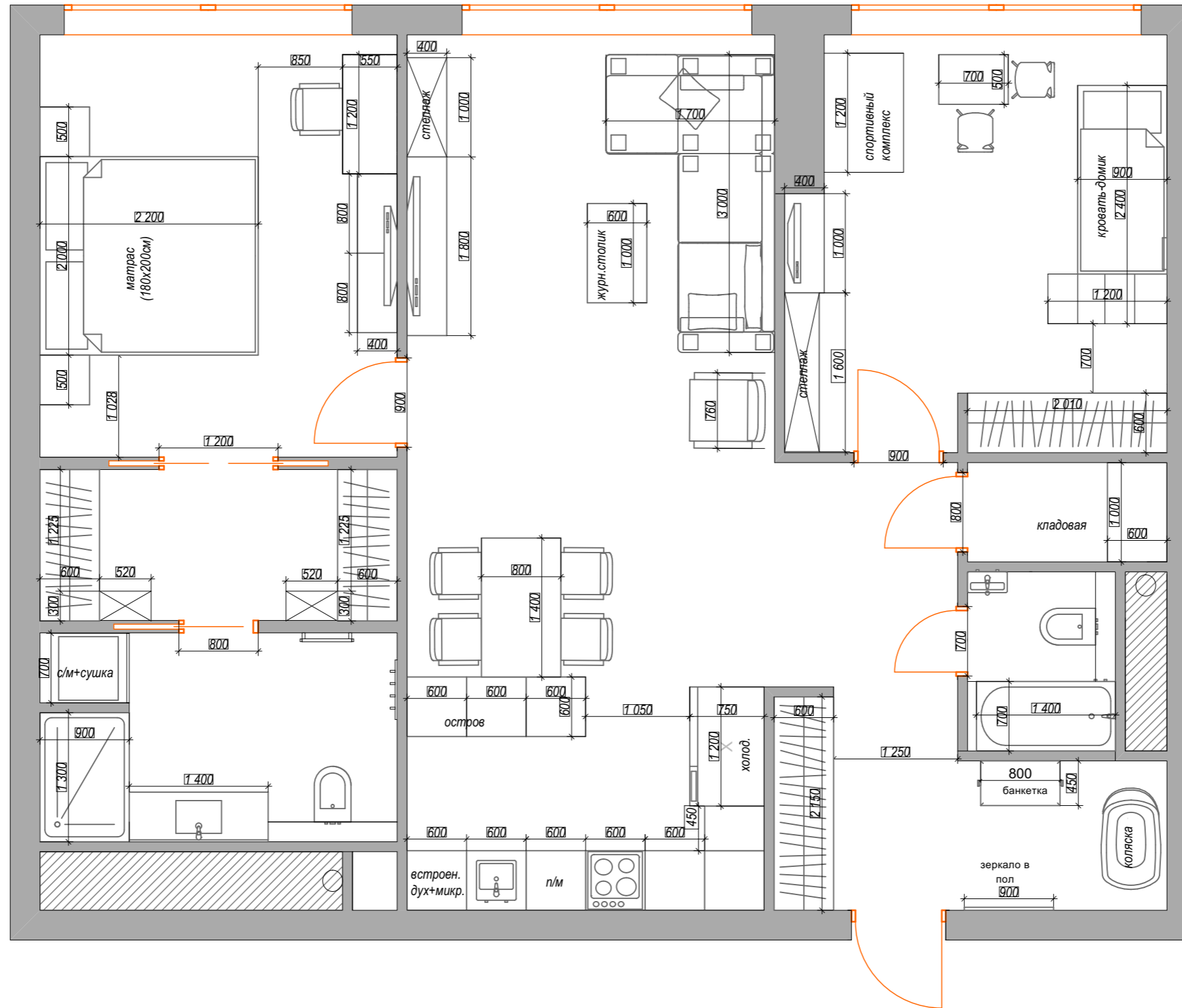
План расстановки мебели. Вариант 2
