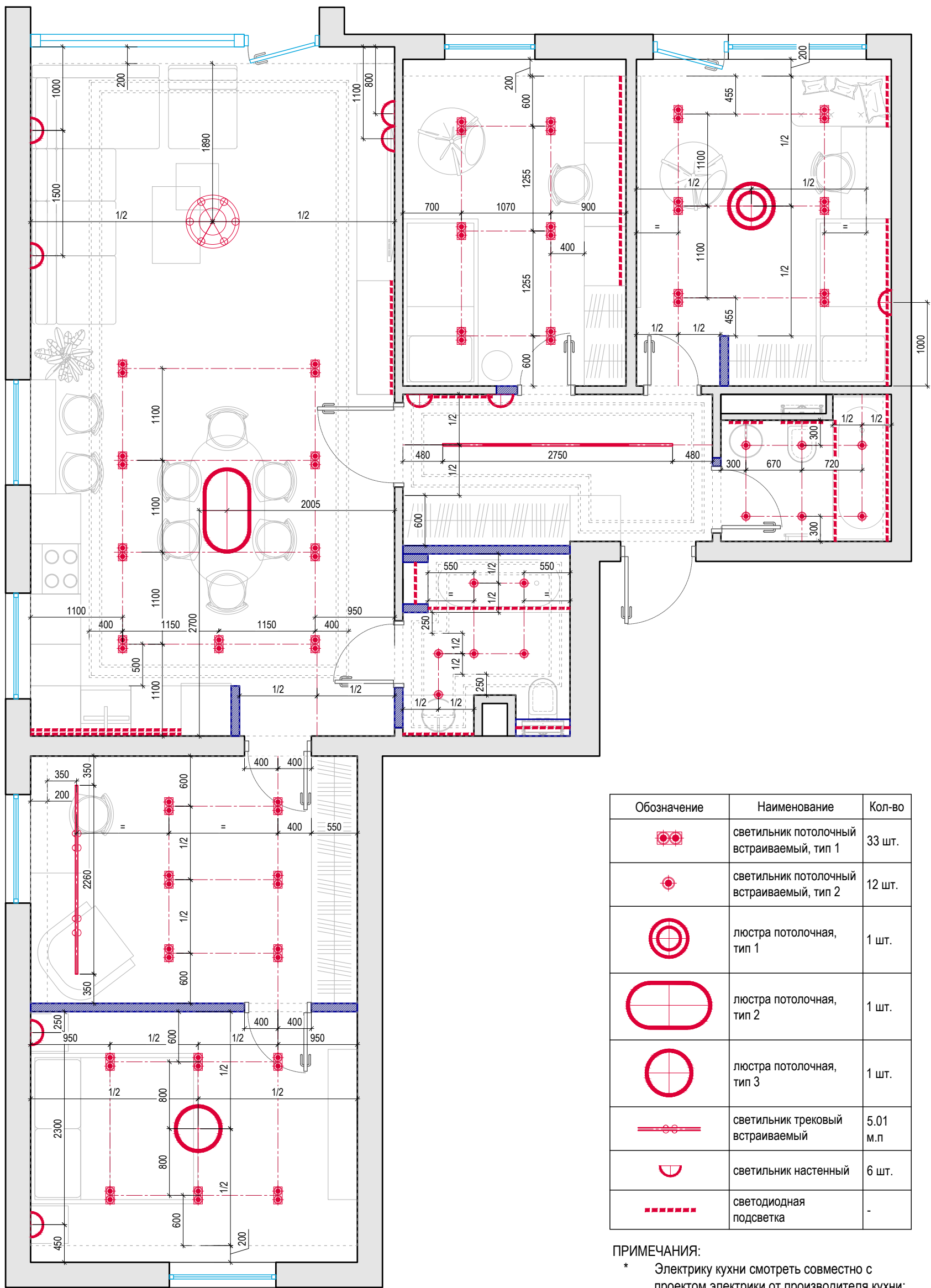
План привязки осветительного оборудования М 1:50
