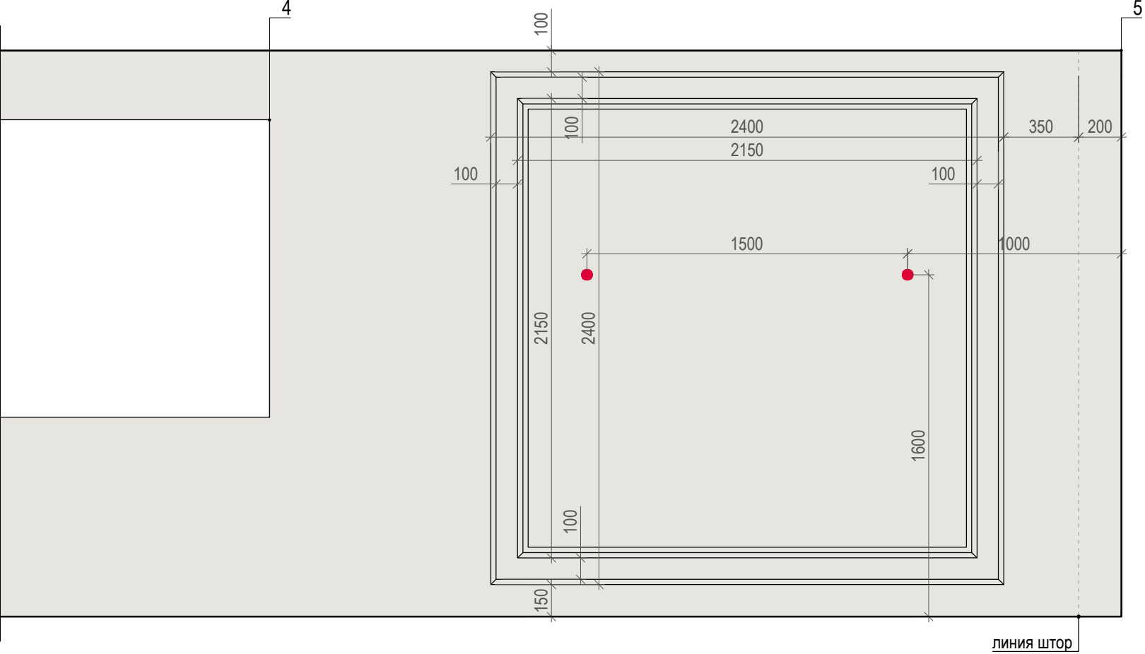
Схема размещения настенных молдингов
