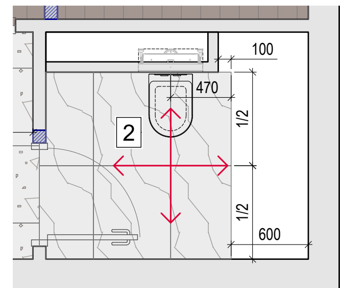
План раскладки напольной плитки
