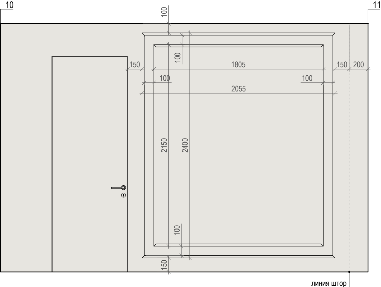
Схема размещения настенных молдингов
