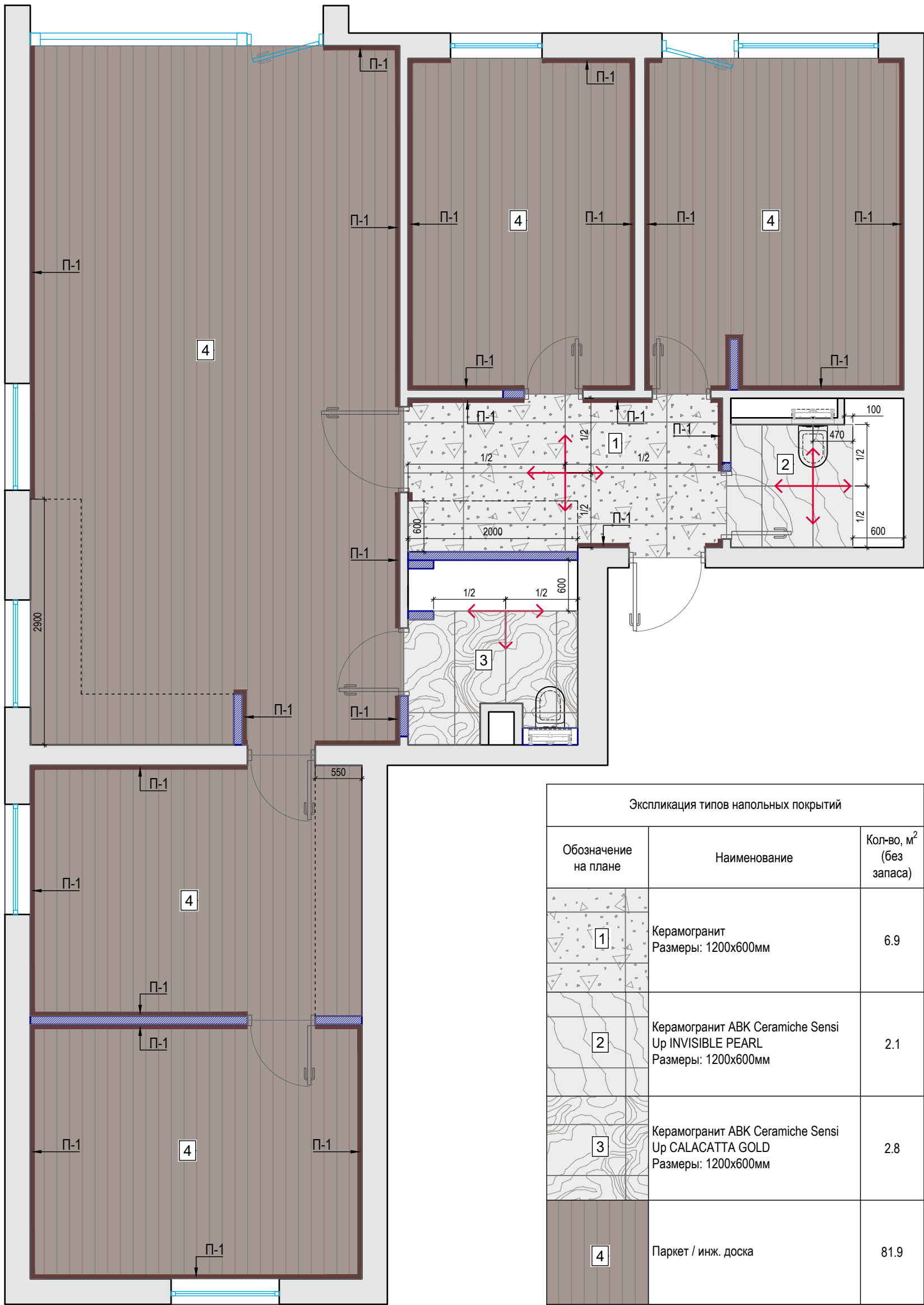
План раскладки напольных покрытий М 1:50
