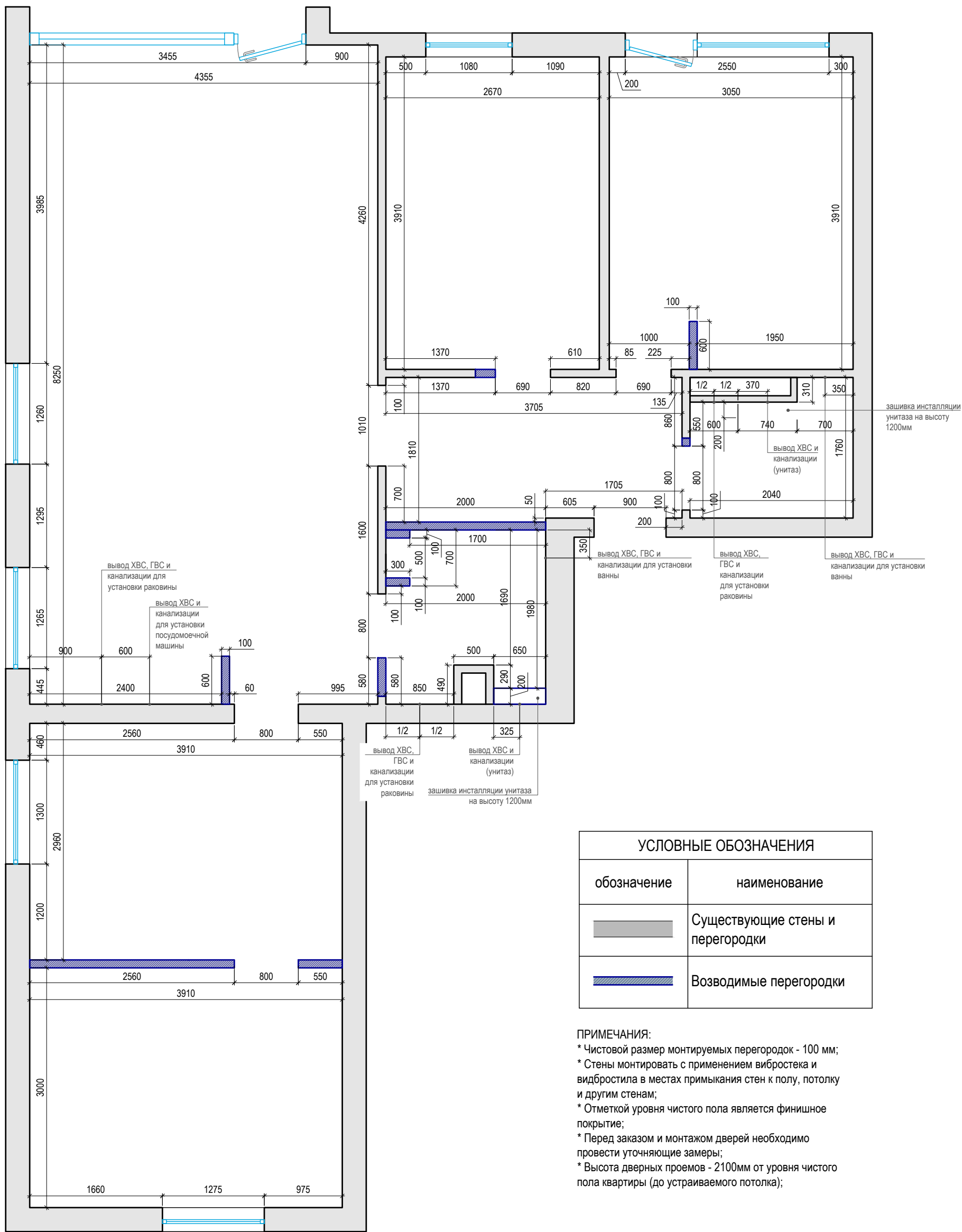
План возводимых перегородок М 1:50
