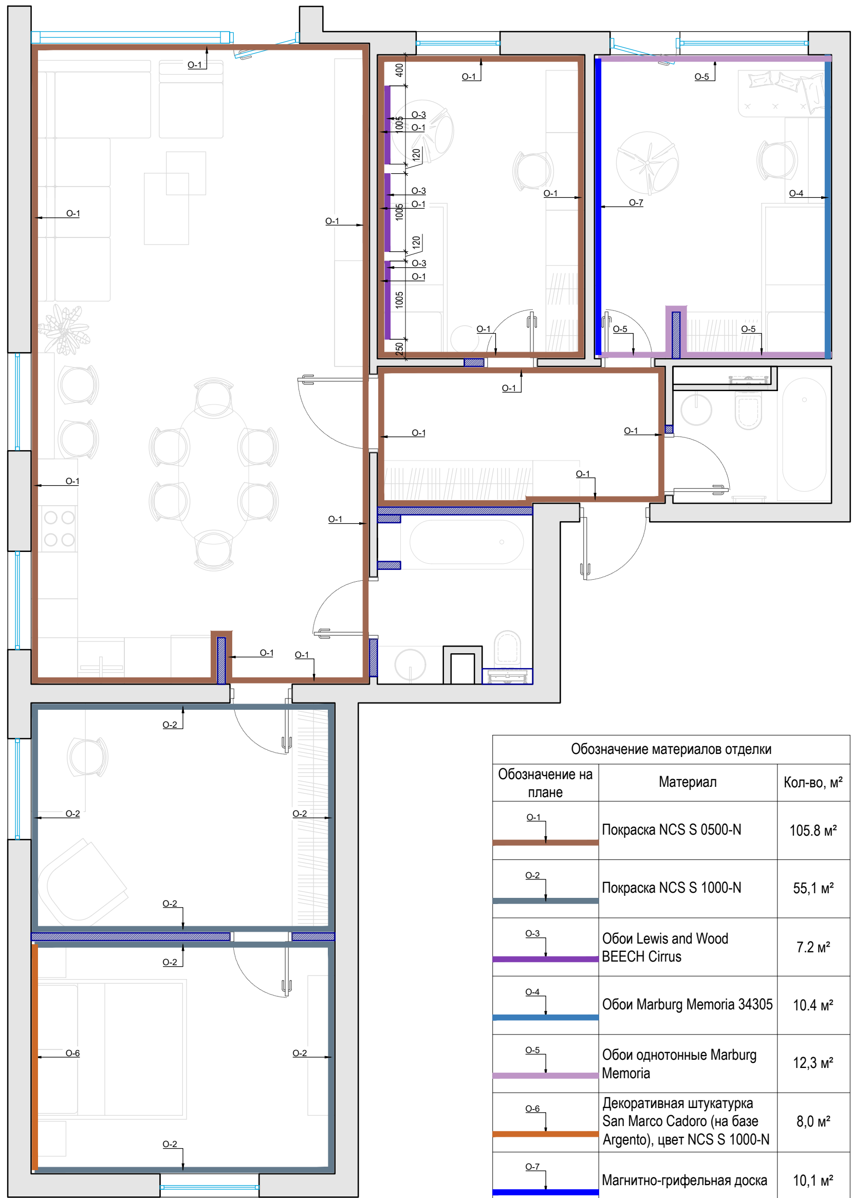
План отделки стен М 1:50
