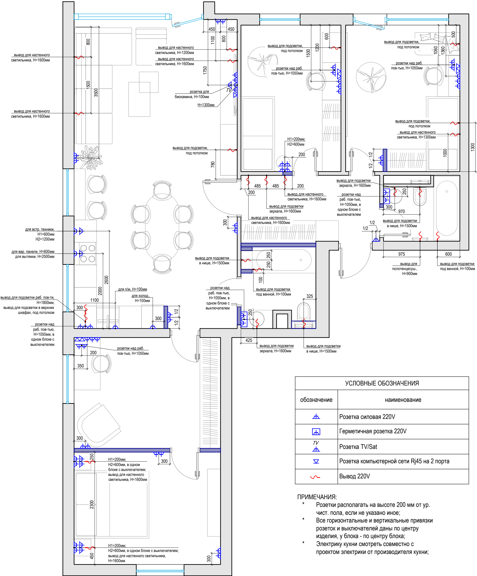
План привязки розеточных групп и электровыводов. М 1:50
