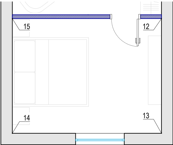
План маяков для разверток стен
