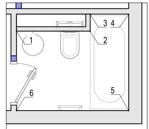
План раскладки напольной плитки
