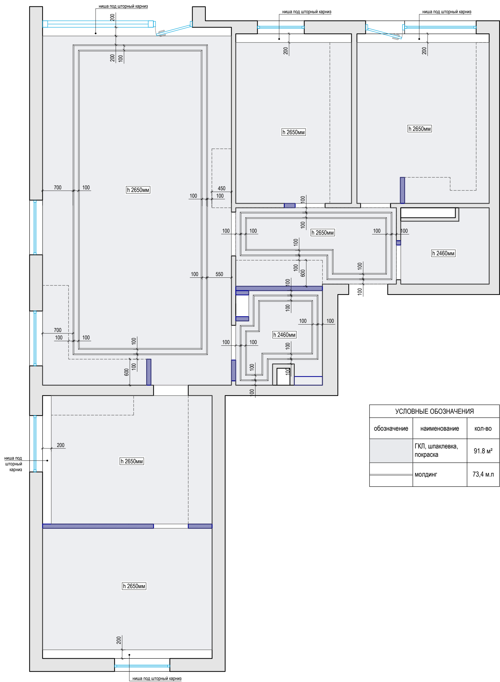
План потолков с указанием высотных отметок. М 1:50
