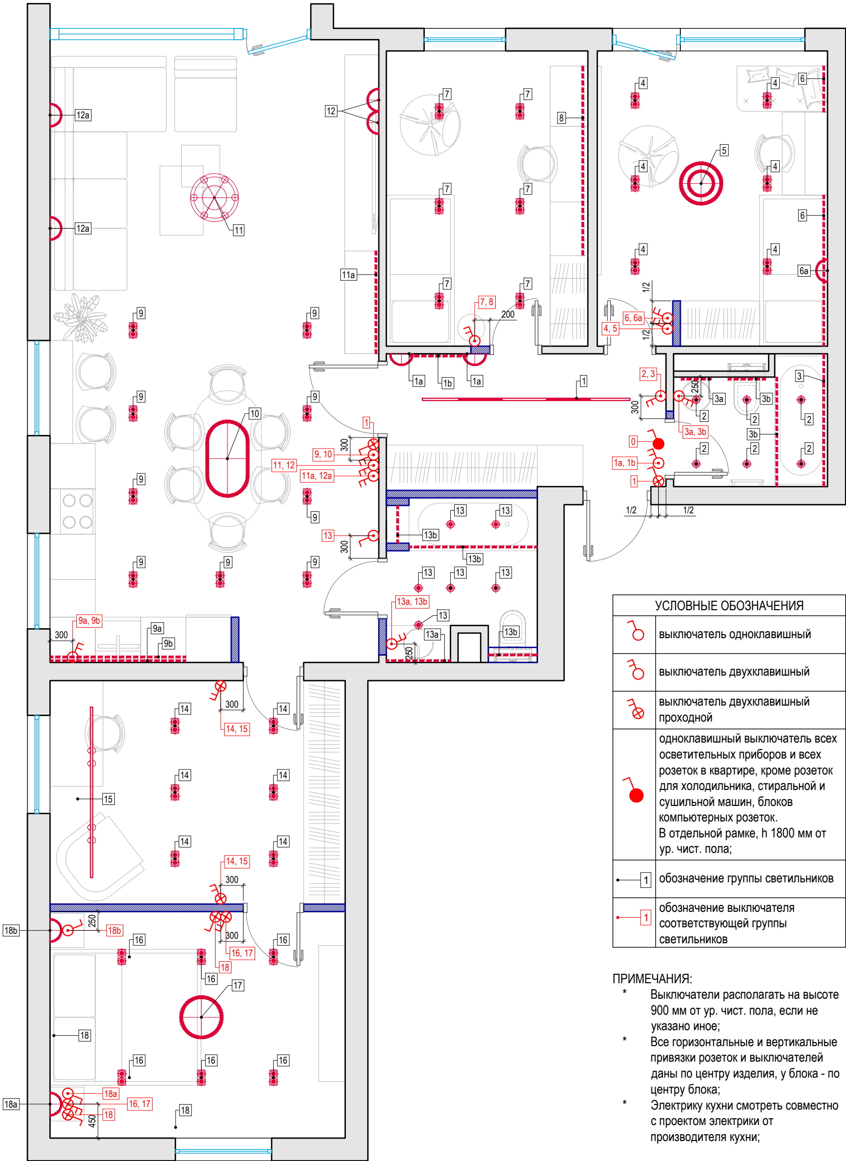
План привязки выключателей с указанием групп включения светильников М 1:50
