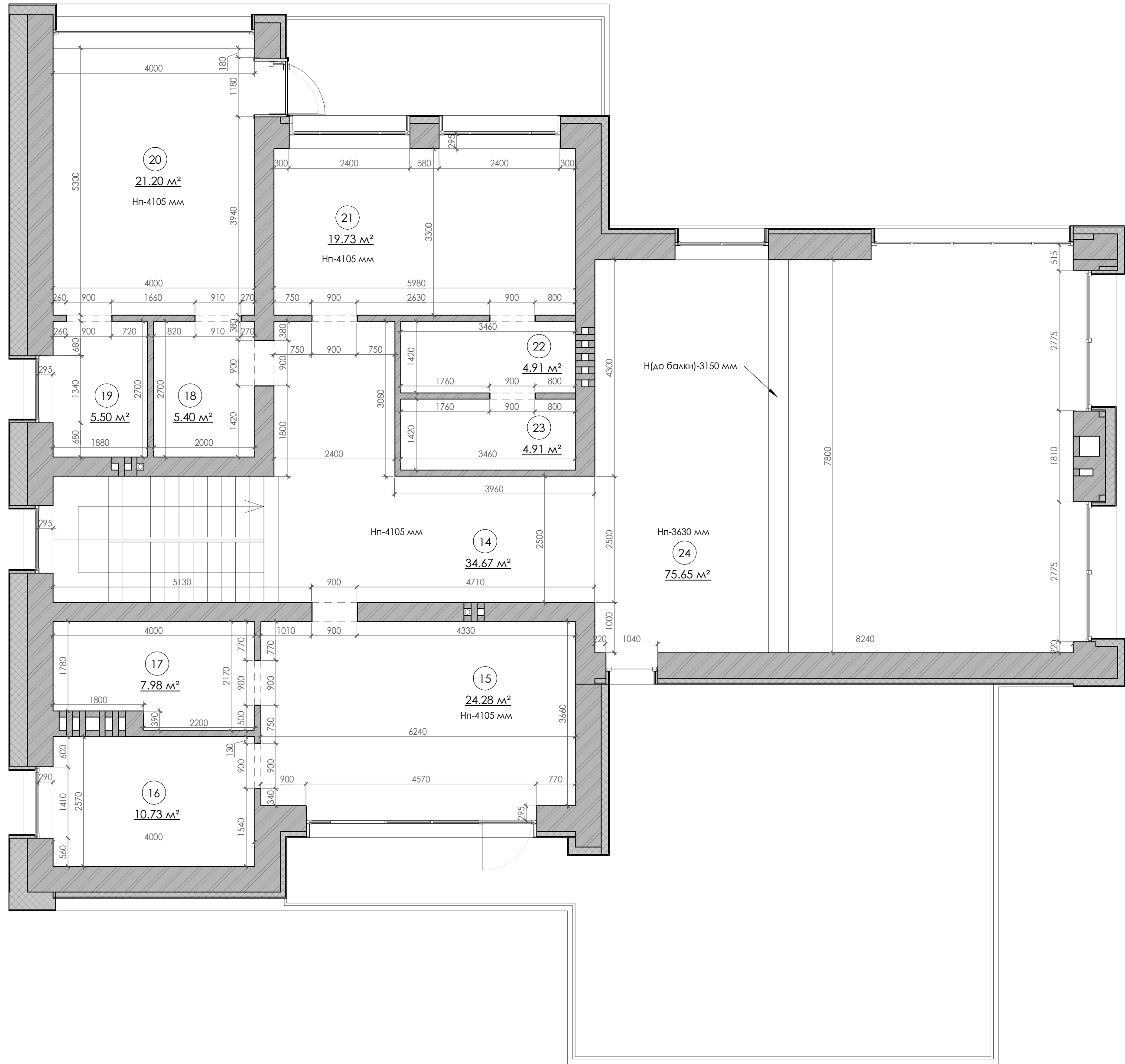
Обмерный план ( 2 этаж) 1 : 65
