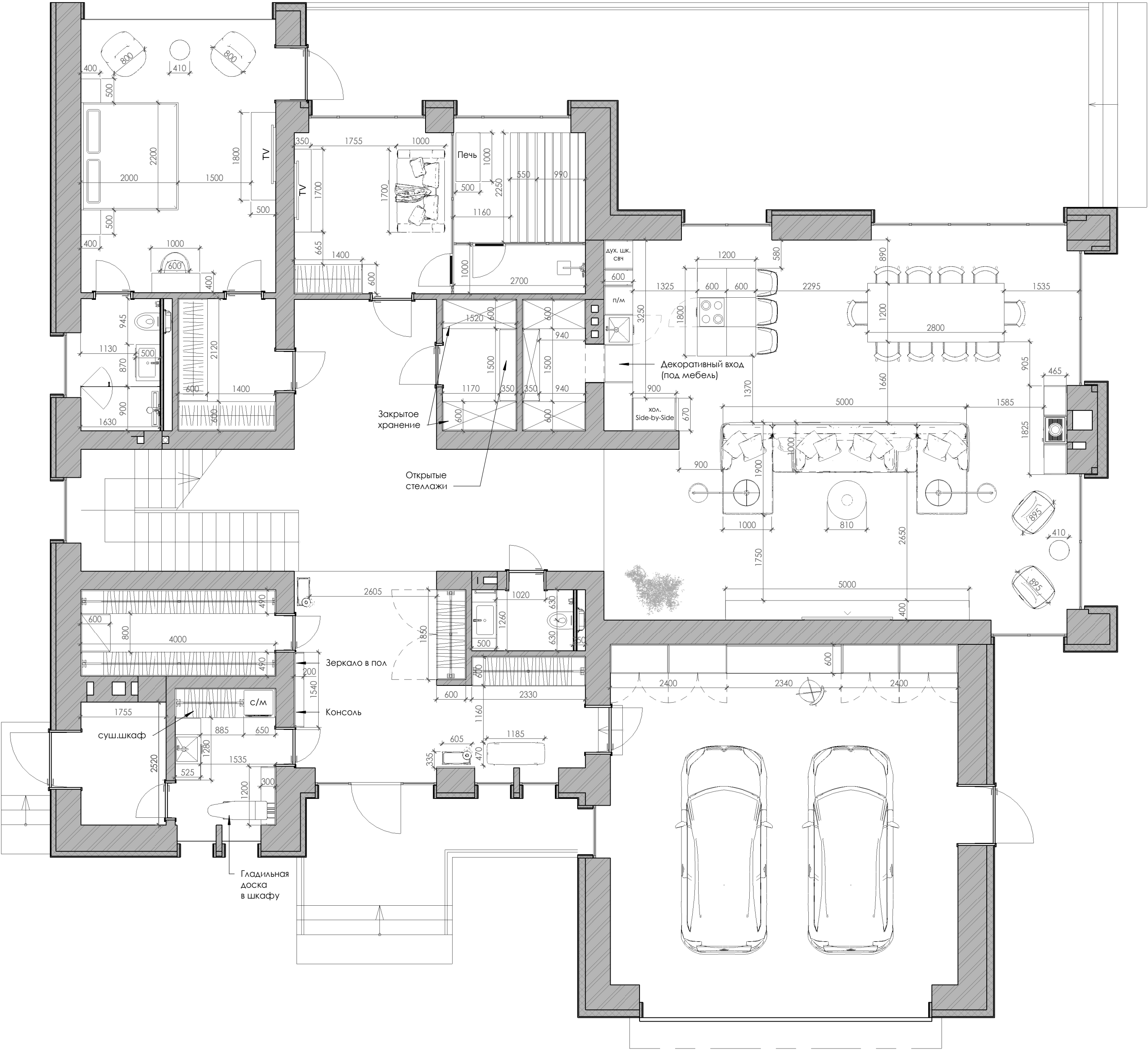
Планировочное решение (1 этаж) 4 в 1 : 65
